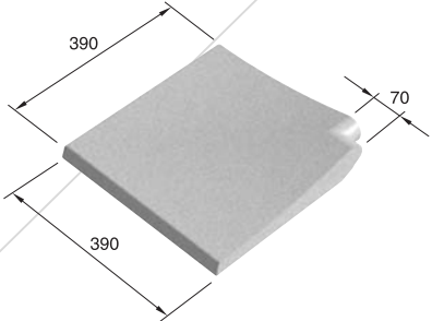
kg 11,5 Angolo retto Right angle Angle droit Randstein estück
